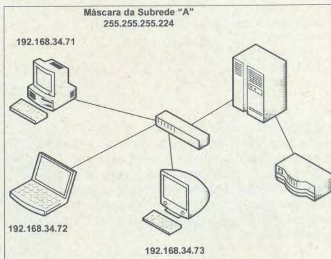
Figura 13 - Rede de computadores
