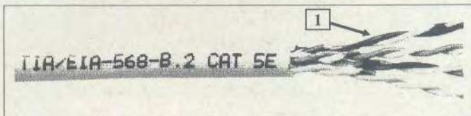
Figura 10(a) - Cabo de rede
