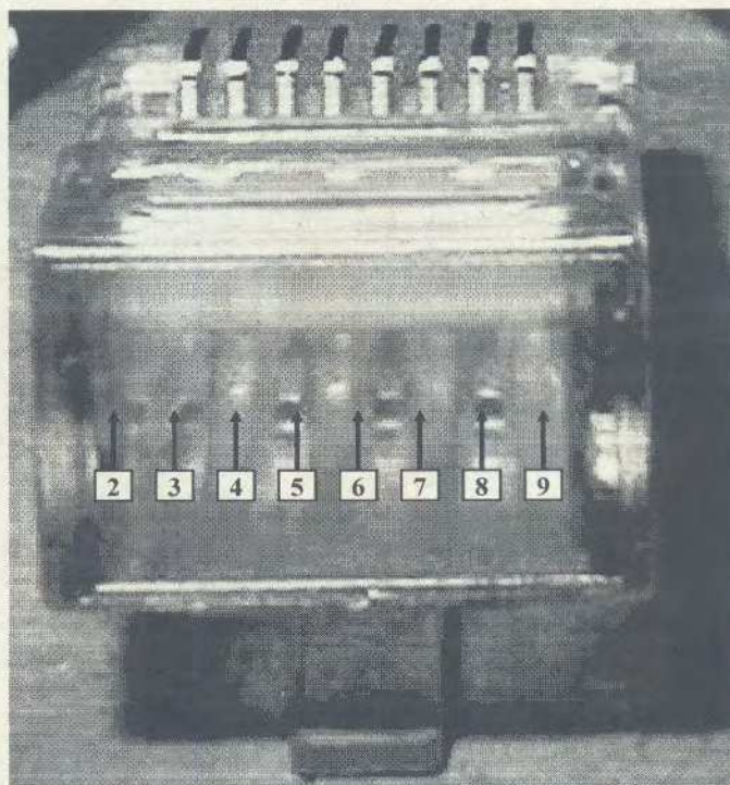
Figura 10(b) - RJ 45 - macho
